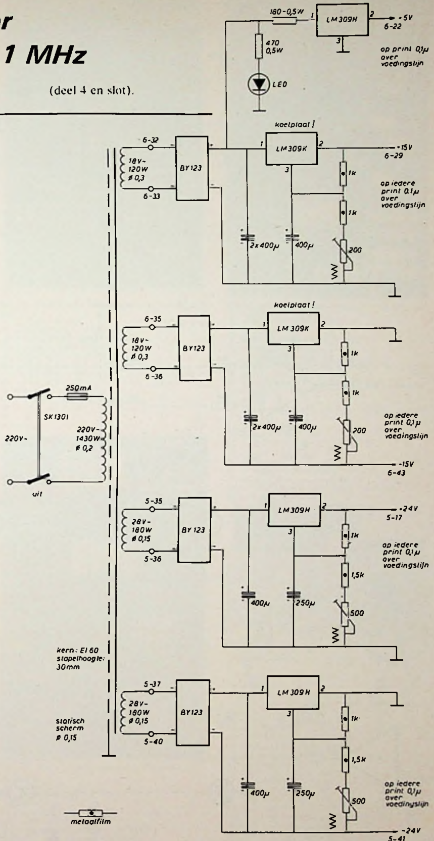
Fig. 13. Voeding-kaart 5 en 6.
